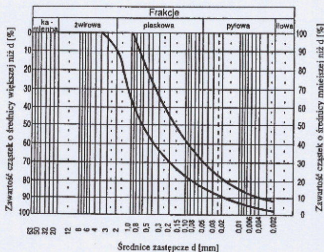
Rys. 1. Obszar uziarnienia optymalnej mieszanki gliniasto-piaskowej
